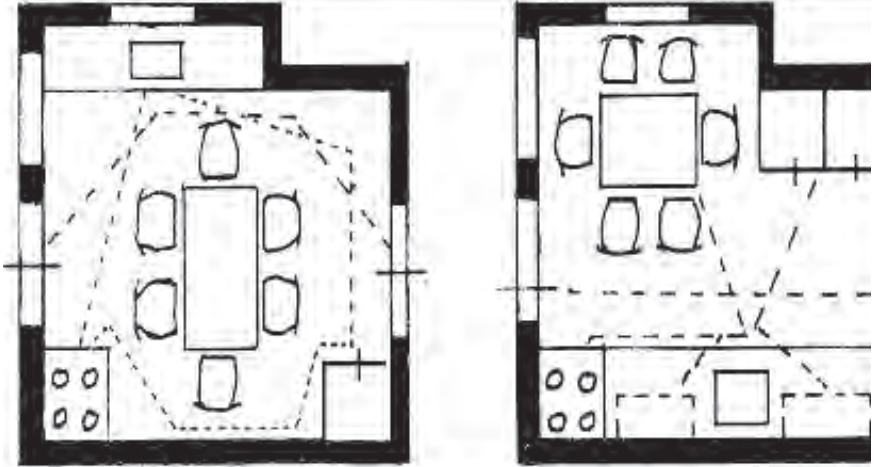
Efficiënte inrichting van een keuken door reductie van looplijnen. Model van de huishoudelijke voorlichting. Uit: Zes jaar streekverbetering Den Ham-Daarle. Ontwikkelingen in de periode 1962-1968 (Hengelo O. 1968) 29.
